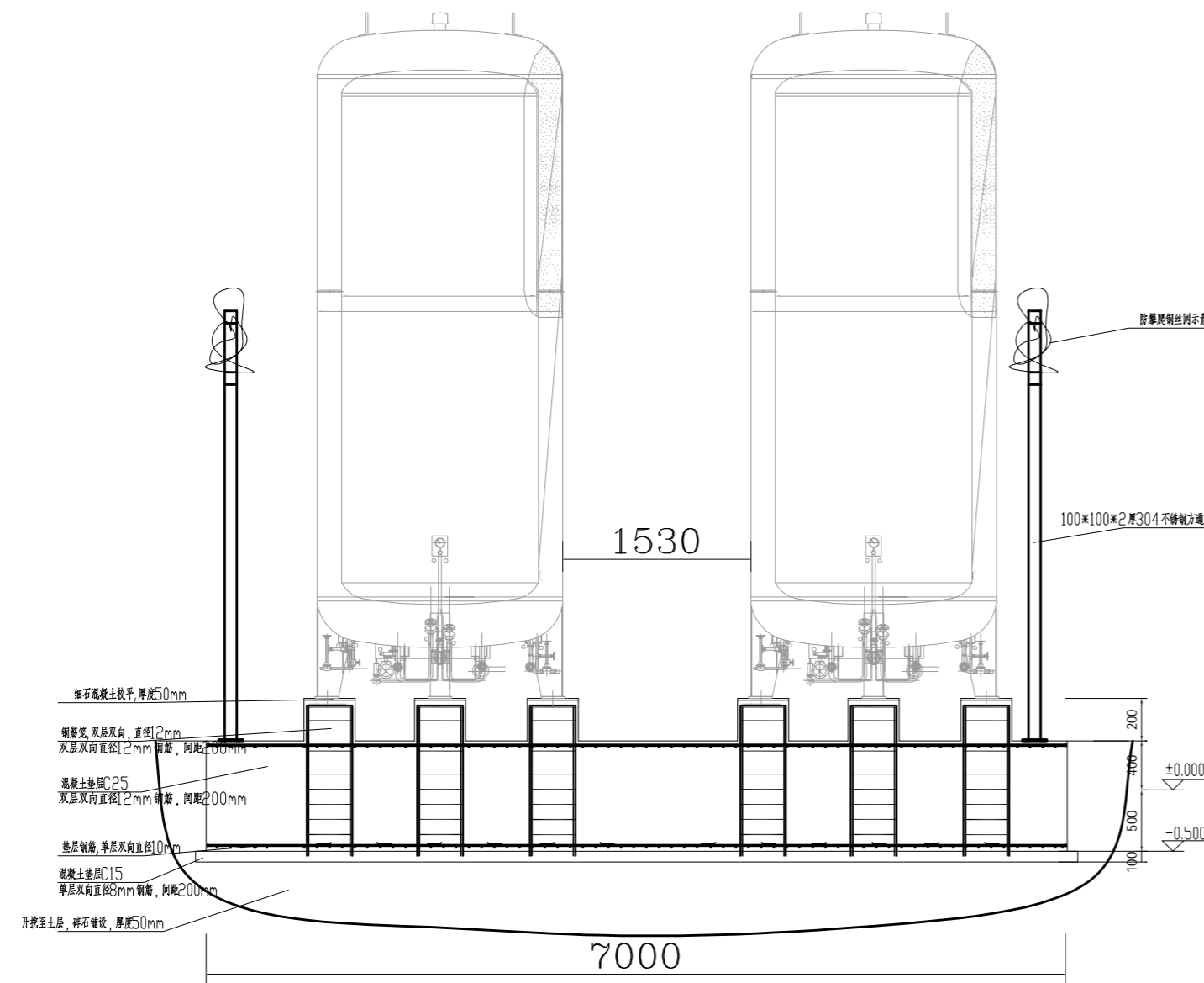
A-A剖面图
