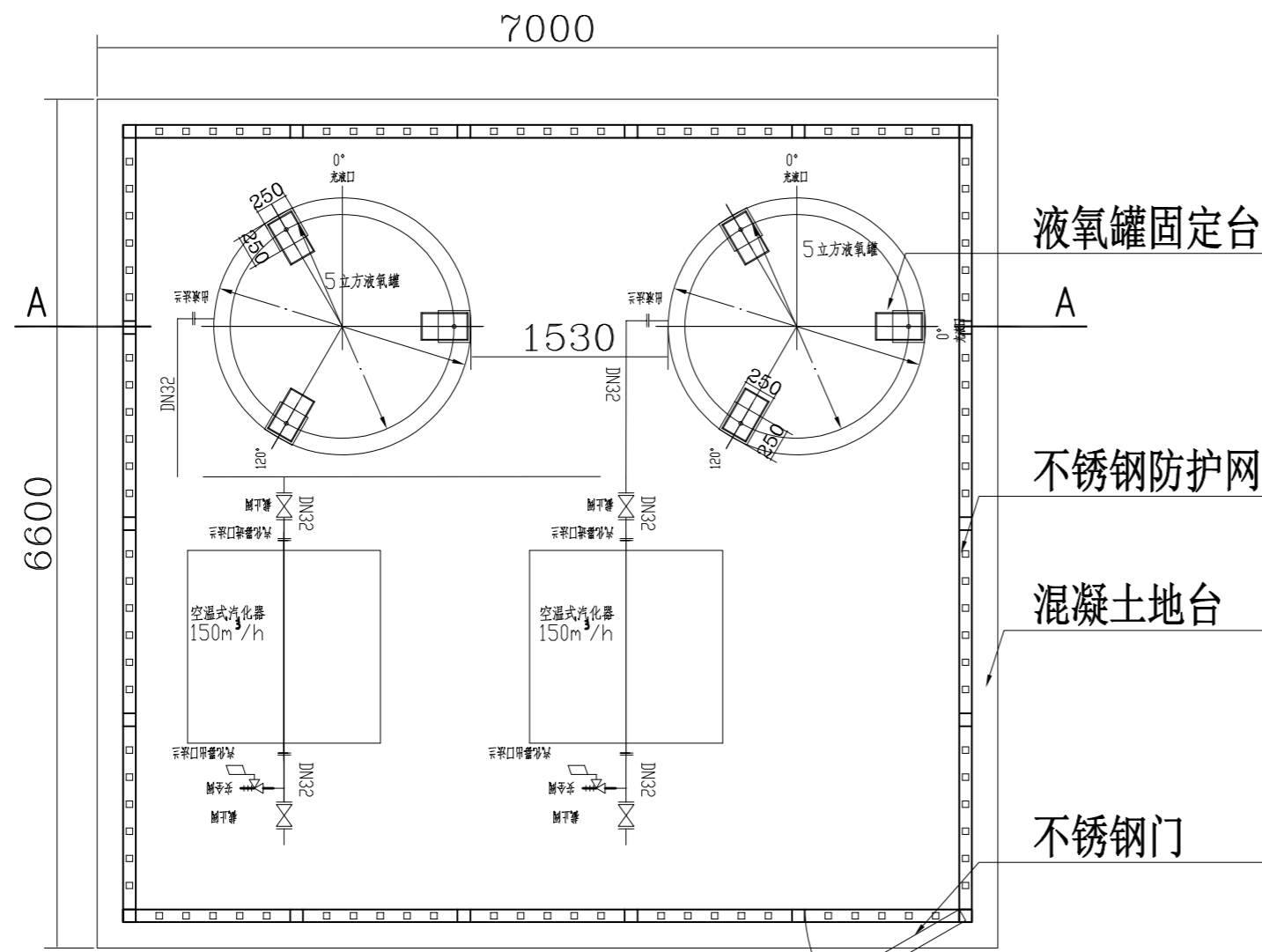
新做地台平面图
