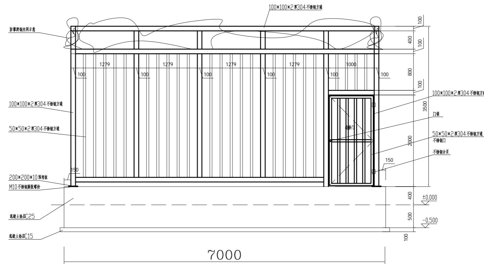
01立面图
