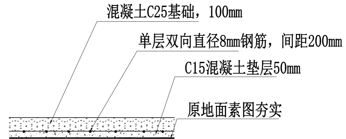
氧气储罐房地面硬化大样图
